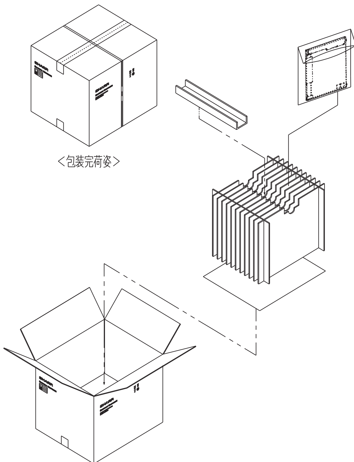
图3. 包装形態図
