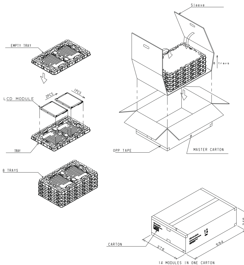
图3 包装形态图
